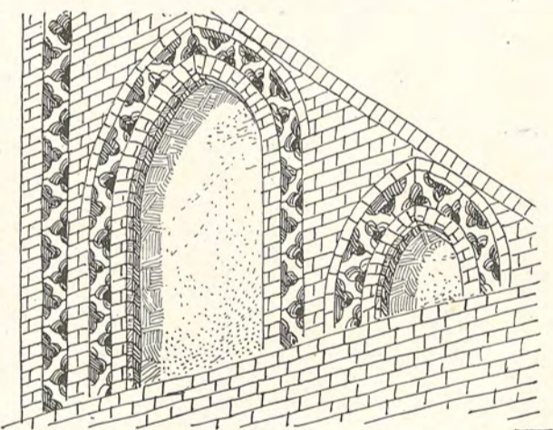
Blenden am Chorgiebel der Petri Kirche zu Stendal 99. G
