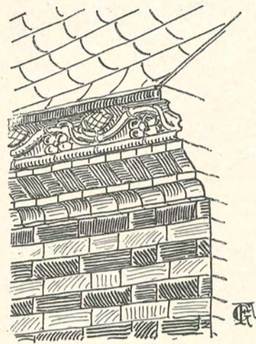
Hauptgesims des Holstenthores zu Lübeck.
